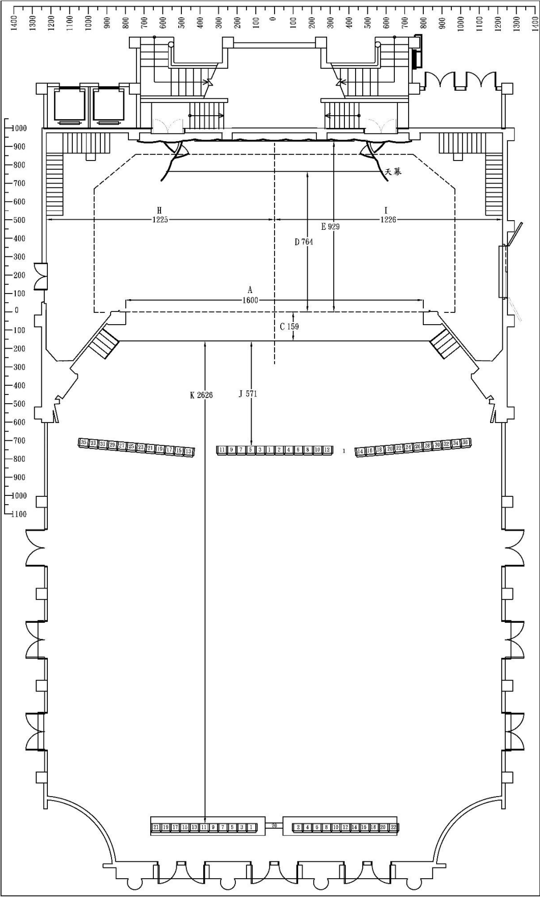
中正廳舞台基本尺寸圖
