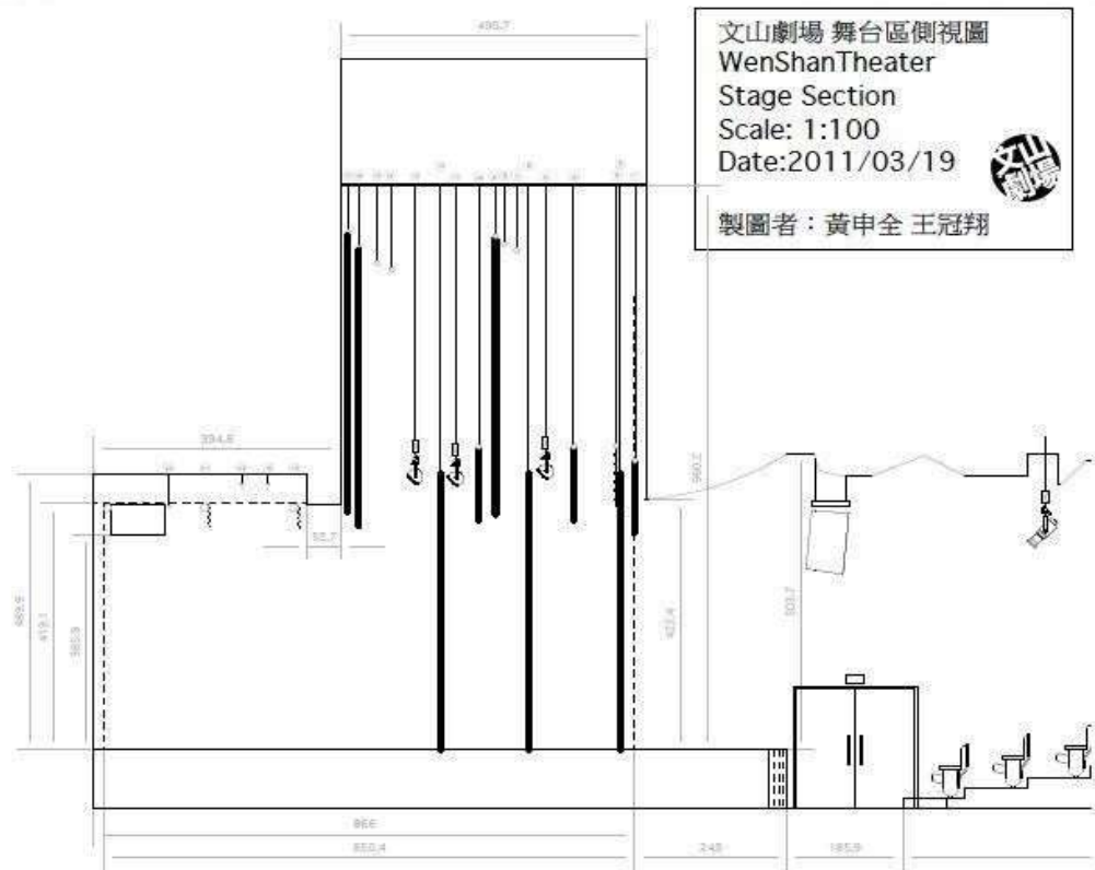
舞台側視圖
